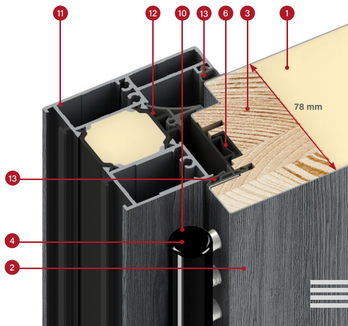
THERMO HOT 78 varčios aliumininės staktos skerspjūvis
