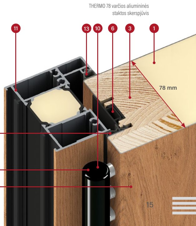
THERMO 78 varčios plieninės staktos skerspjūvis
