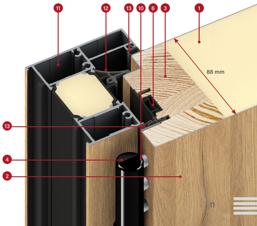
THERMO HOT 88 varčios aliumininė staktos skerspjūvis
