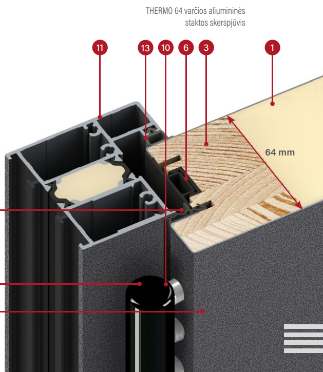
THERMO 64 varčios plieninės staktos skerspjūvis
